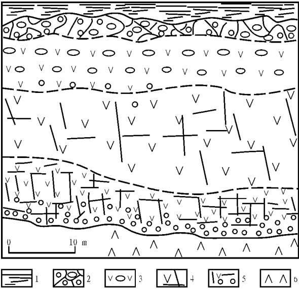
图 4 徐家围子断陷营城组火山岩岩层序
