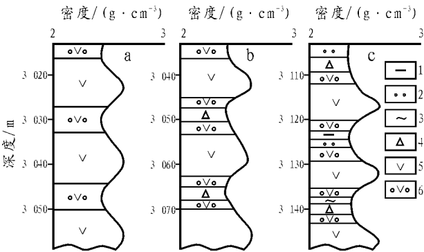
图 2 徐家围子断陷营城组火山岩组合类型
