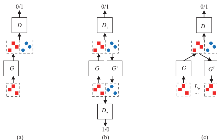
图6 (网络版彩图) 对抗学习
