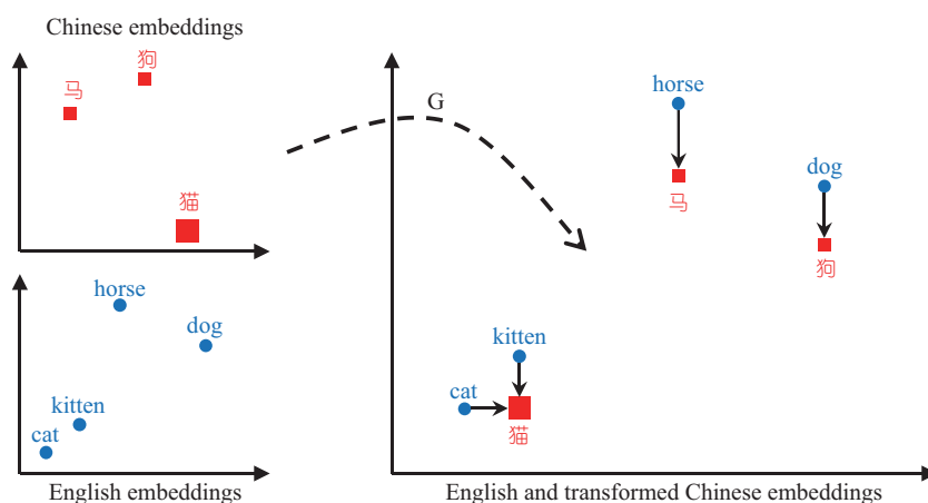
图 7 (网络版彩图) Earth mover's distance 最小化学习
