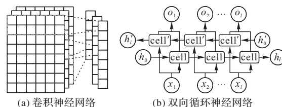
图1 序列特征提取方法
