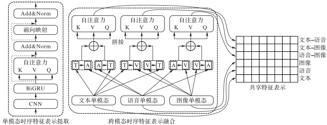
图3 上游特征表示模型结构
