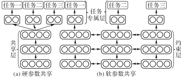
图2 多任务学习的参数共享机制
