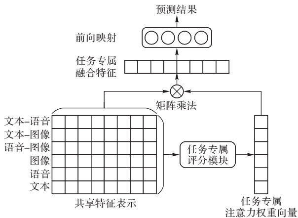
图6 任务专属特征融合
