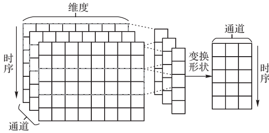
图4 卷积神经网络提取局部时序信息
