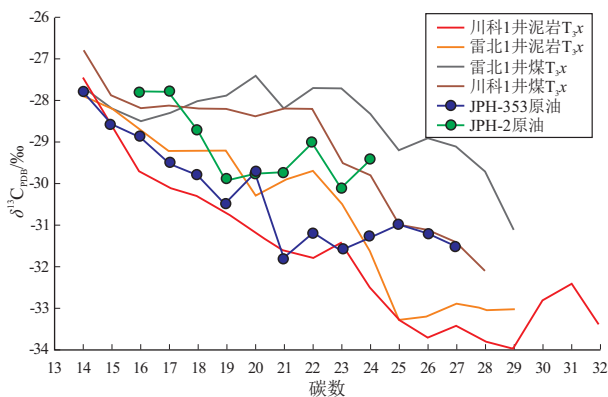
图 5 鄂尔多斯盆地杭锦旗地区 上古生界原油正构烷烃单体碳同位素分布曲线 川科 1 井和雷北 1 井数据引自文献[27]。
