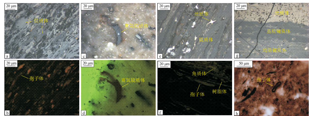
图6 鄂尔多斯盆地杭锦旗地区上古生界烃源岩有机岩石学照片 a-b.J116井,3 064.4 m, P_1s^1 ,煤;c-d.J78井,3 108.98 m, P_1s^2 ,煤;e-f.J35井,2 167.7 m, P_1s^2 ,碳质泥岩;g.J70井,2 976.43 m, C_3t ,煤;h.Y18井, P_1s ,煤
