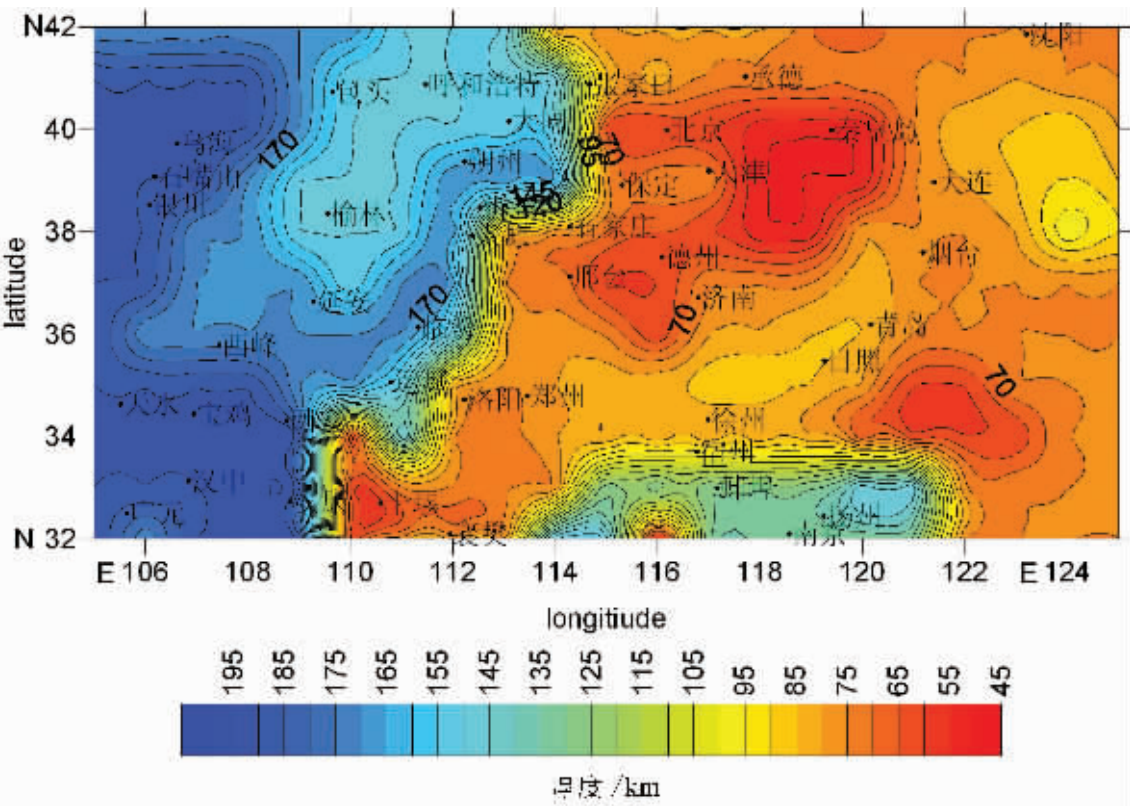
图 7 岩石圈等厚度图
