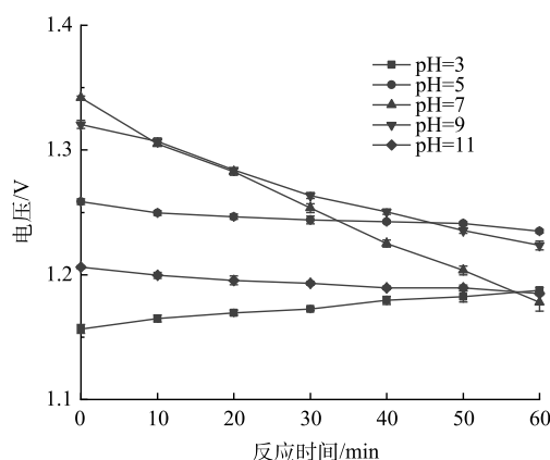
(a) 极板间电压
