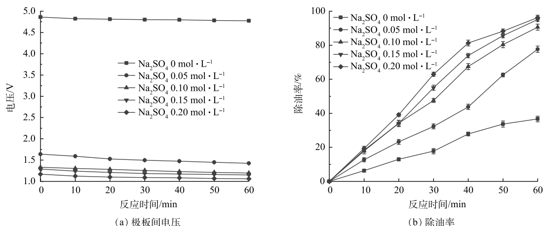
图 4 不同支撑电解质浓度下, 极板间电压及除油率随反应时间的变化
