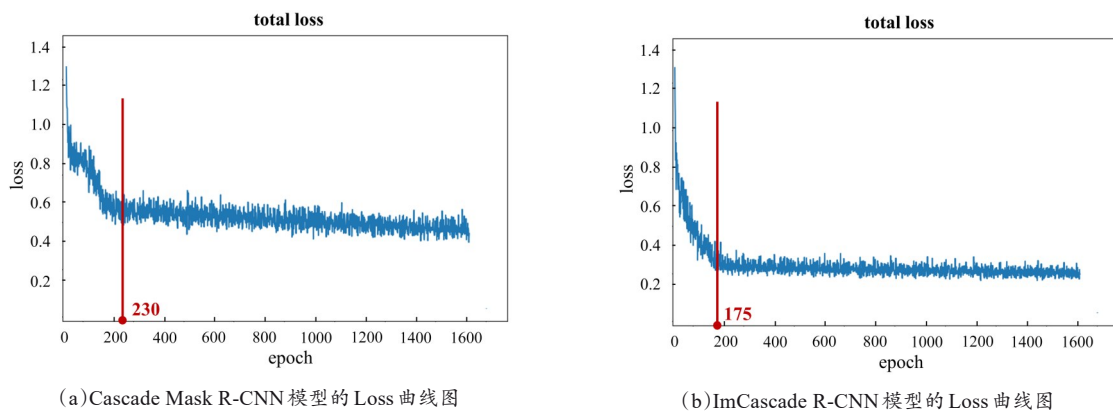
图 11 籽粒识别、分割实验的 Cascade Mask R-CNN 模型与 ImCascade R-CNN 模型的 Loss 曲线图
