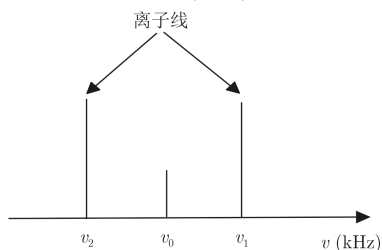
图1 离子谱图
