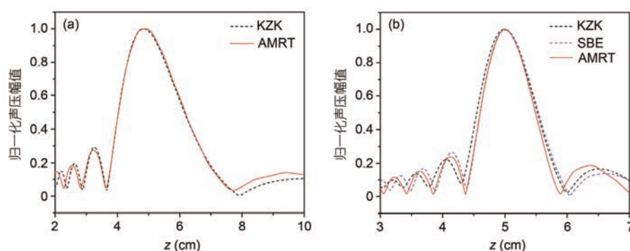
图2 (网络版彩色)归一化轴向声压幅值分布. (a) W=4 cm; (b) W=6 cm
