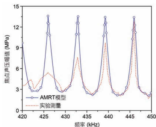
图3 (网络版彩色)焦点声压幅值随频率变化
