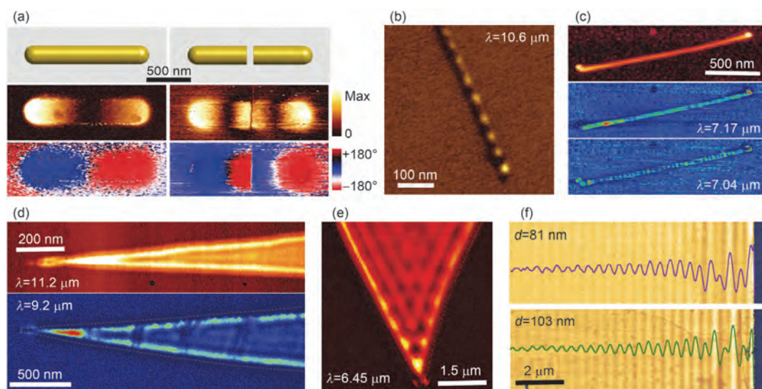
图5 s-SNOM对低维纳米材料/结构本征电磁模式成像. (a) 红外天线 [67] ; (b) 碳纳米管 [68] ; (c) 氮化硼纳米管 [69] ; (d) 石墨烯 [71,72] ; (e) 氮化硼 [73] ; (f) 二硫化钼 [77]
