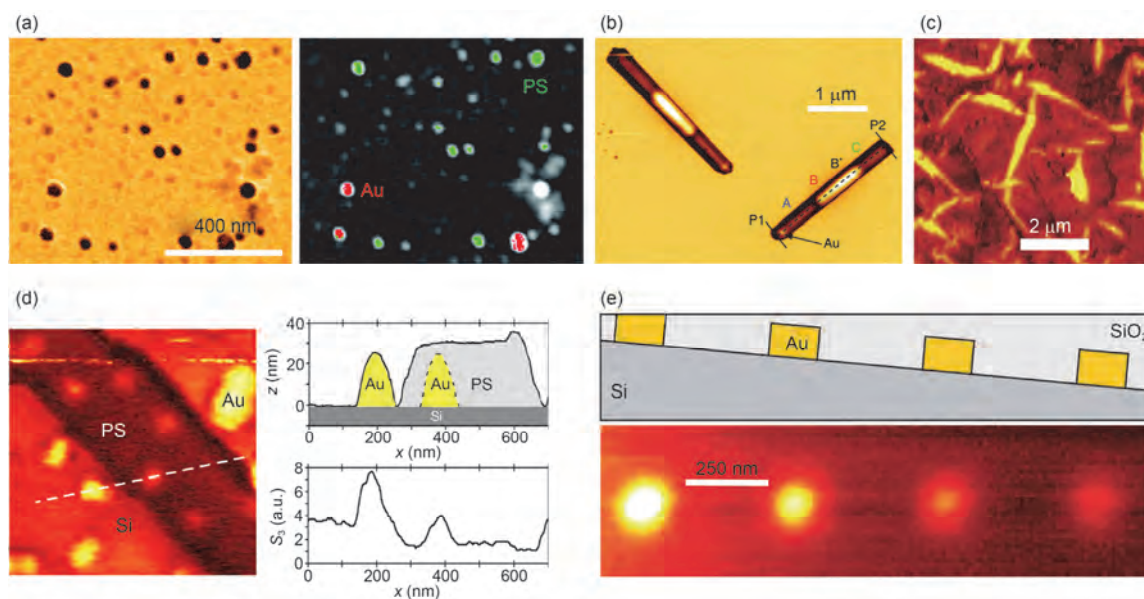
图3 s-SNOM对非均相材料介电常数分布的成像。(a) 纳米颗粒 [53] ；(b) 纳米线 [54] ；(c) 纳米薄膜 [55] ；(d), (e) 亚表面金属纳米结构 [56,57]
