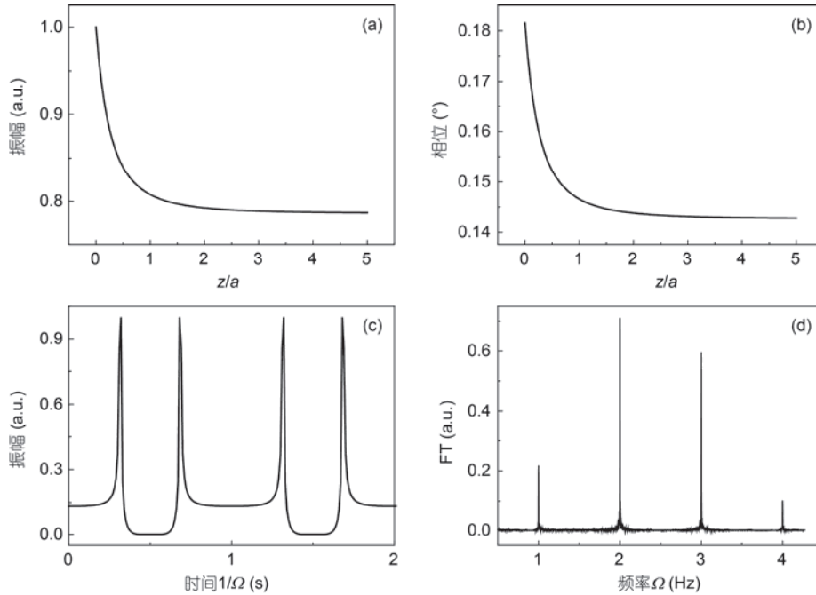
图2 近场信号调制-解调原理. (a), (b) 近场信号振幅及相位与探针-样品距离 z 的关系; (c) 以频率 \Omega 及振幅 a 对 z 进行正弦调制时近场信号振幅随时间的变化; (d) 对(c)进行傅里叶变换得到近场信号在探针调制频率 \Omega 各阶泛频的分量
