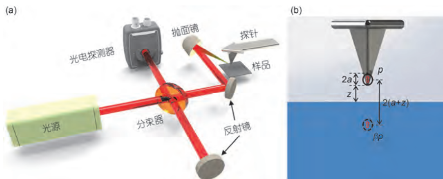
图1 s-SNOM工作原理. (a) s-SNOM结构图; (b) 近场探针与样品相互作用的偶极模型
