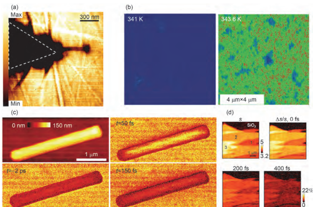
图4 外界条件调控下低维纳米材料介电常数分布近场成像。(a) 应力 [58] ；(b) 温度 [59] ；(c), (d) 光泵浦 [60,61]
