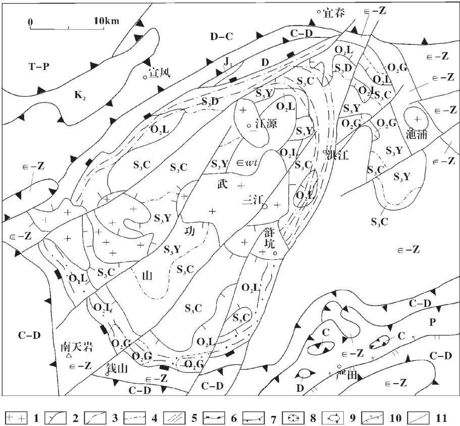
图 1 武功山超单元和洪江超单元平面分布略图
