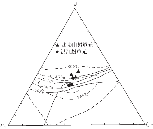
图 4 武功山花岗岩各单元标准矿物 Q-Ab-Or 与结晶时 p-t 关系图
