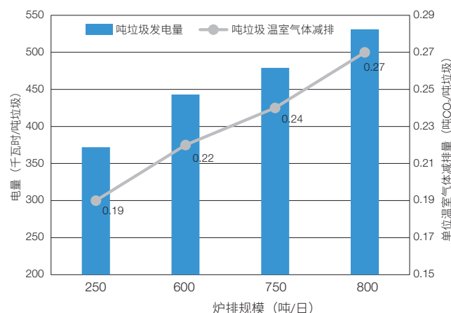
图 4 不同单排炉排规模碳减排量对比 [8,13,14]
