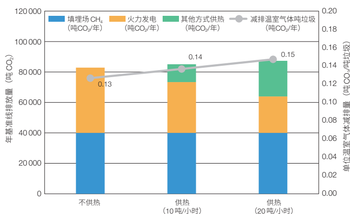
图6 某生活垃圾焚烧厂热电联产基准线碳排放量和碳减排量 [8,13,14]
