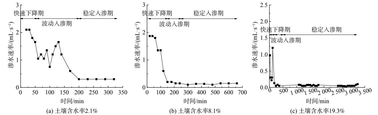
图 5 不同土壤含水率下凹式绿地瞬时渗水速率
