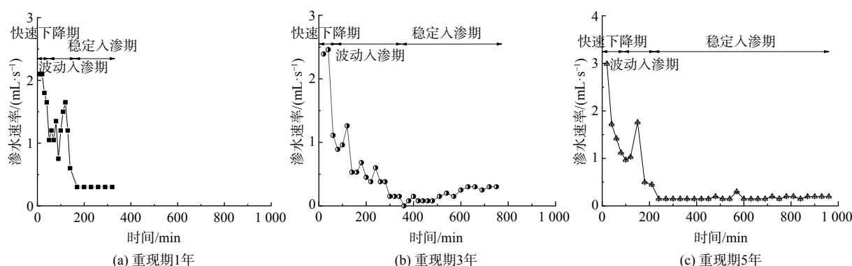
图 4 不同降雨强度下凹式绿地瞬时渗水速率 (降雨历时: 120 min)
