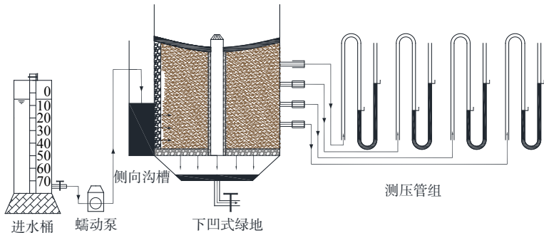
图 1 模拟下凹式绿地反应装置图 Fig. 1 Simulated concave green space reaction device
