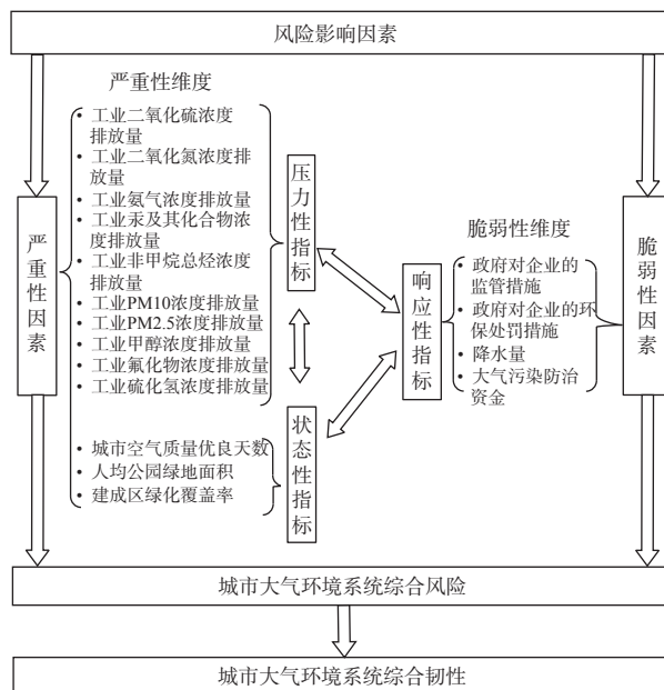
图 2 基于 RMA-PSR 模型的城市大气环境系统韧性评价机理图
