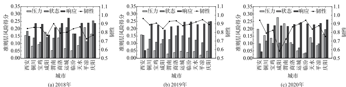
图 5 2018—2020 年关中城市群各城市大气环境系统各准则层及韧性得分
