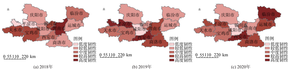
图6 2018—2020年关中城市群城市大气环境系统韧性空间格局演化图
