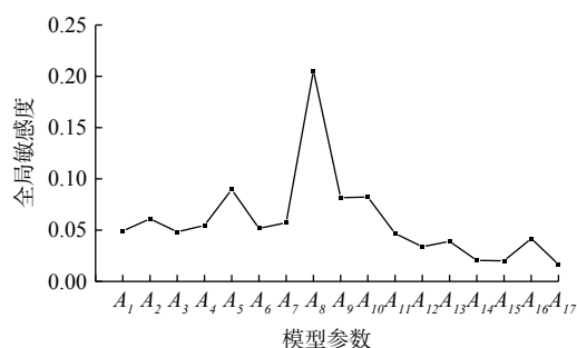
图 4 RMA-PSR 模型全局敏感度指标
