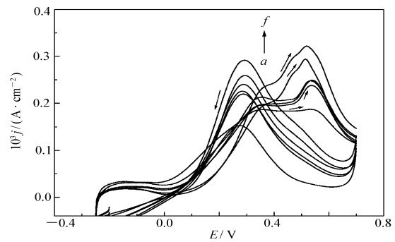
图 4 EG 在不同 PtSn/P 电极上的 CV 曲线
