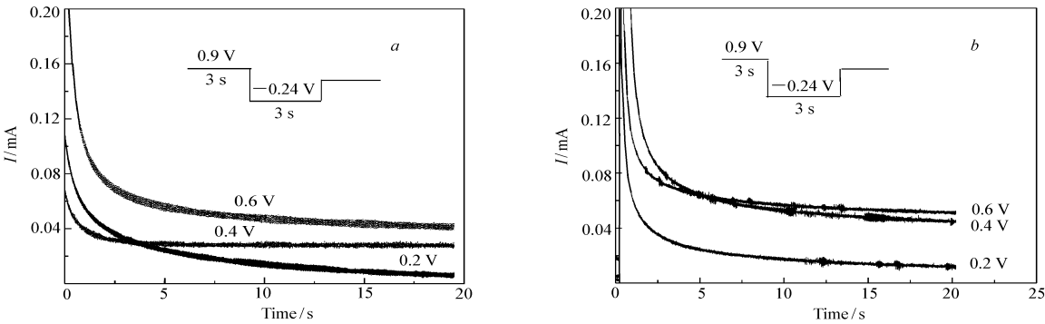
图 5 EG在 Pt/P(a)和 PtSn/P(b)电极上的计时电流曲线
