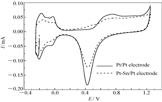
图 1 PtSn/P 和 Pt/Pt 电极于 0.1 mol/L H_2SO_4 溶液中的循环伏安曲线
