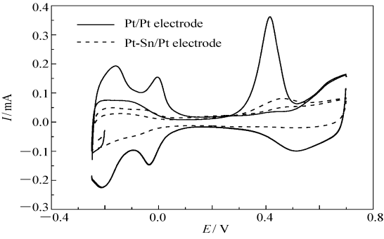
图 2 Pt/Pt 和 PtSn/P 电极浸于 0.1 mol/L EG + 0.1 mol/L H_2SO_4 溶液 3 min 后的 CV 曲线
