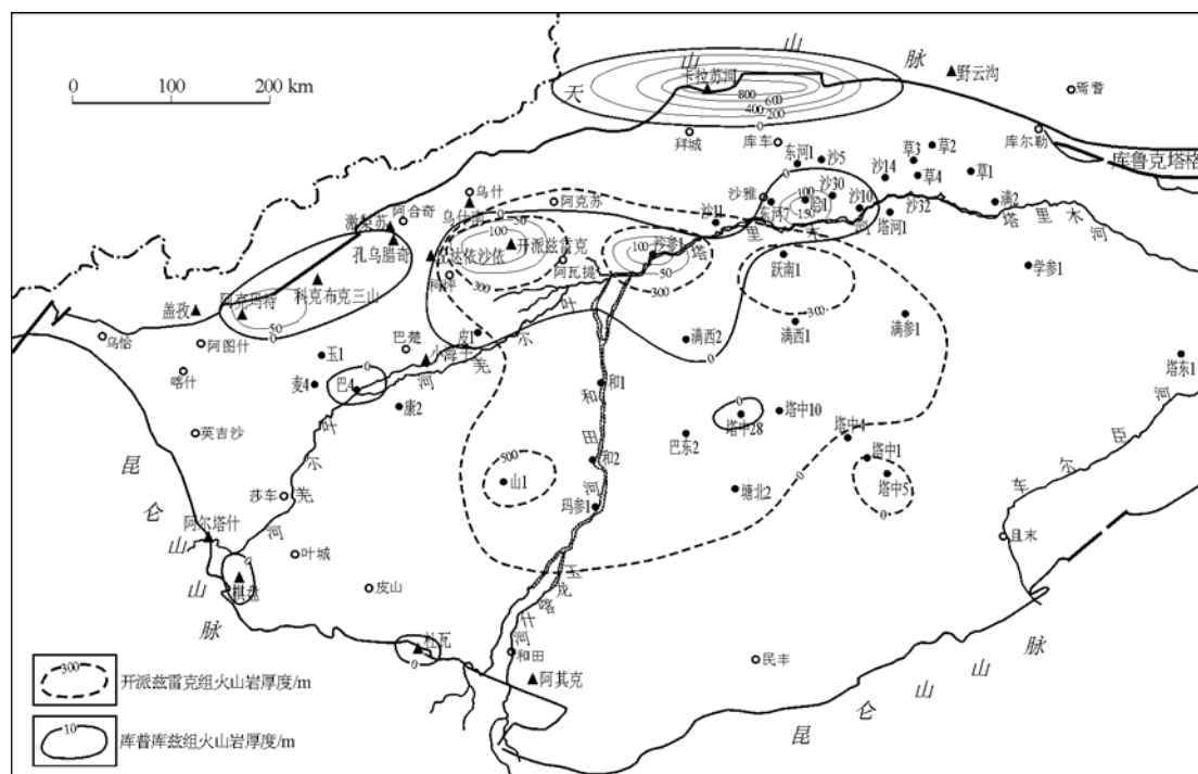
图1 塔里木盆地二叠统火山岩分布
