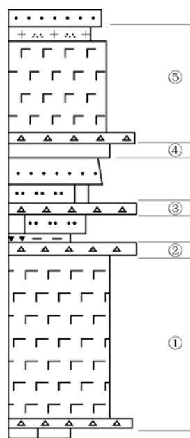
图2 塔里木盆地开派兹雷克剖面 下火山岩段旋回结构示意图 圆圈内数字为火山喷发旋回编号
