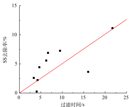
图6 过滤时间对SS去除率的影响
