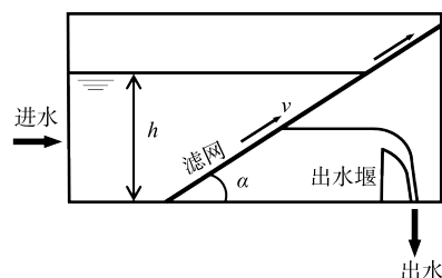
图5 旋转式带式过滤器结构示意图
