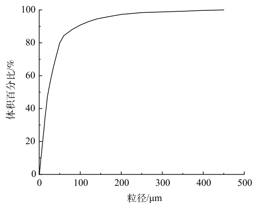
图2 进水颗粒物体积累积分布
