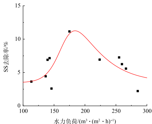
图7 水力负荷对 SS 去除率的影响
