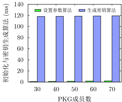
图 6 初始化与密钥生成阶段的执行时间
