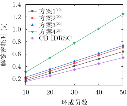
图 4 解签密耗时比较
