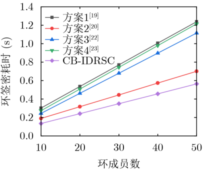
图 3 环签密耗时比较图
