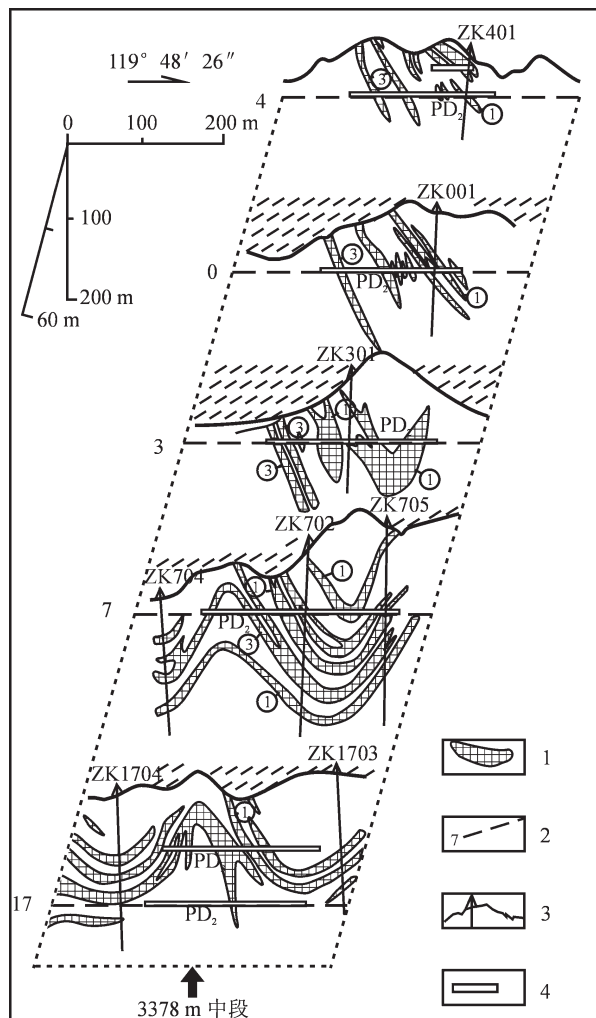
图6 滩间山金矿床4至17勘探线①号和③号矿体3维空间分布略图(据青海第一地质大队资料编制)
