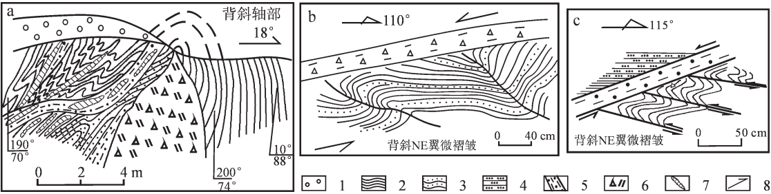
图 4 3~18 号矿体控矿背斜素描图
