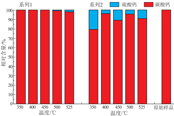
图 3 模拟实验固体产物中不同含钙化合物拟合结果 Fig. 3 Fitting results of calcium entities of samples
