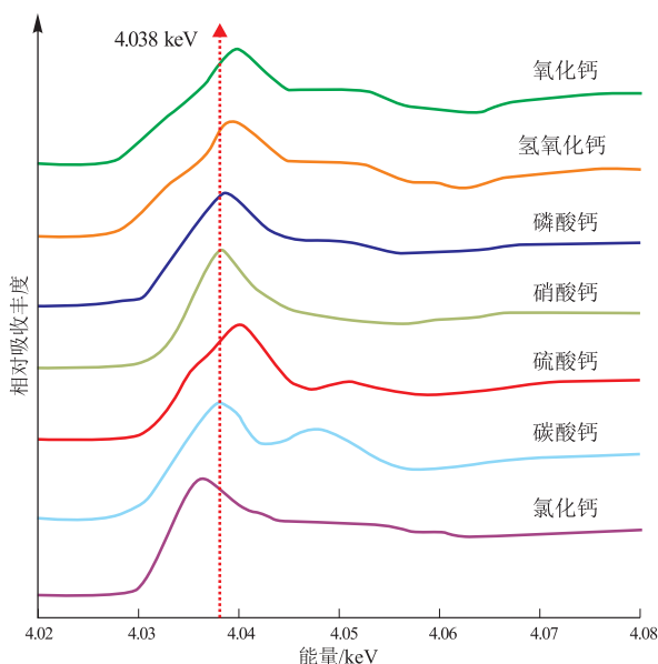
图 1 含钙标准化化合物样品的 K 边 XANES 谱
