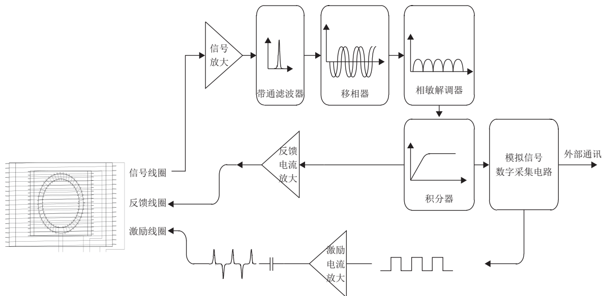
图1 磁通门磁强计工作原理图
