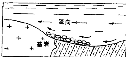
图 6 谷底低洼处对金粒阻留示意图
