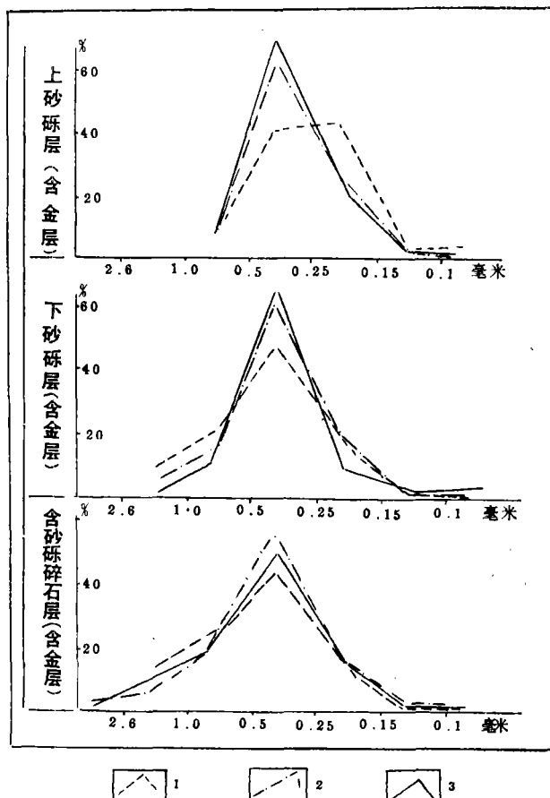
图 8 吉韩矿区 1 号砂金矿体含金粒度变化曲线图 1—上游砂金粒度变化曲线，2—中游砂金粒度变化曲线， 3—下游砂金粒度变化曲线
