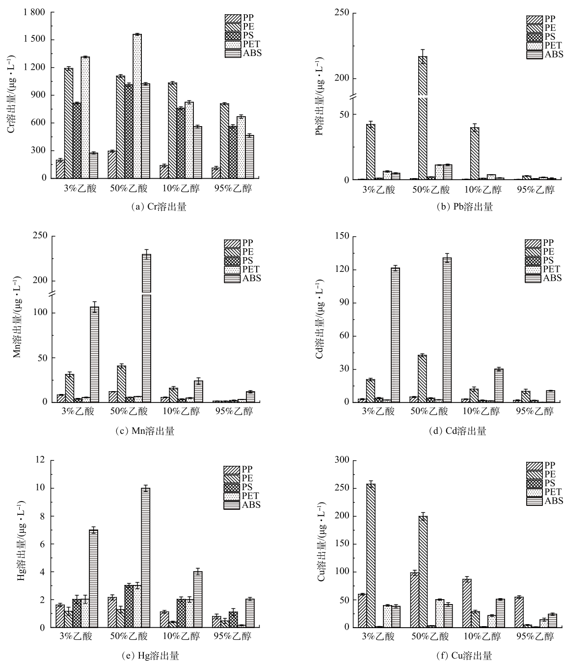
图3 5种再生塑料颗粒中的6种重金属在25℃下向不同食物模拟液中的溶出量
