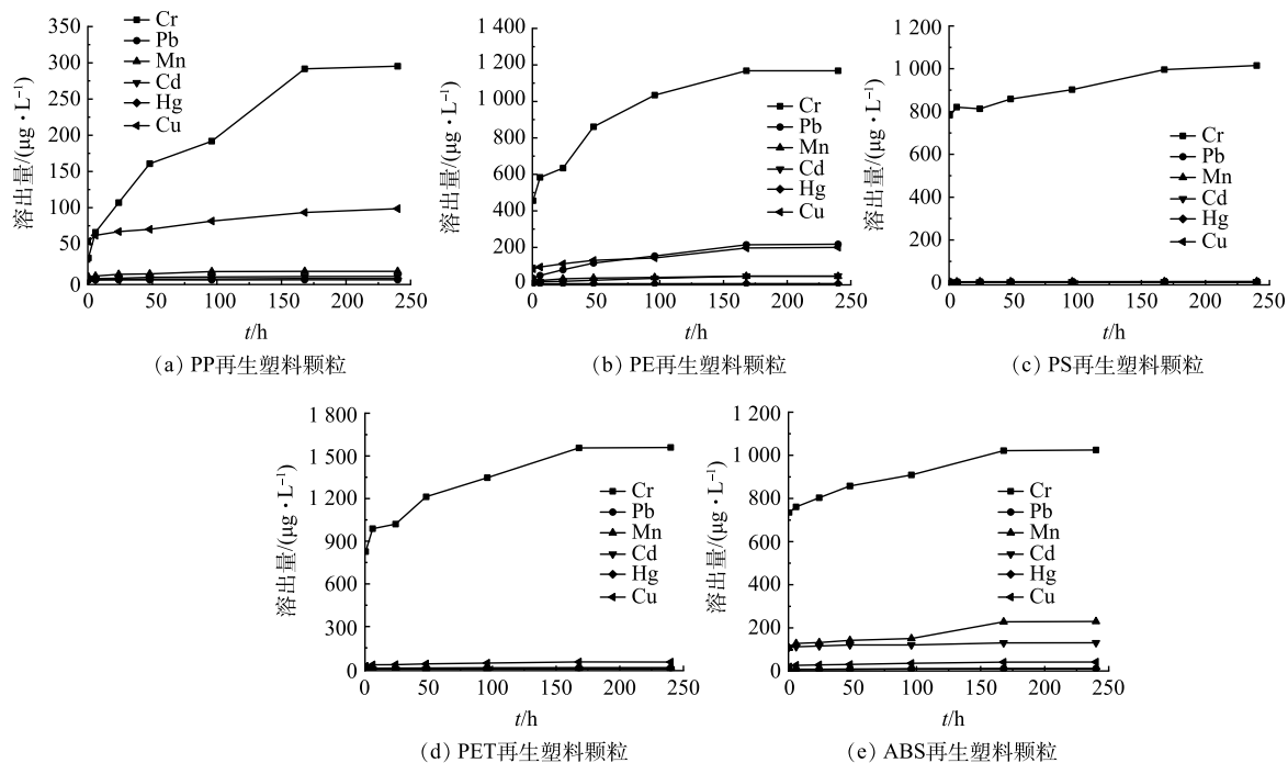
图 2 25 °C 下 5 种再生塑料颗粒中重金属在 50% 乙酸条件下的溶出曲线
