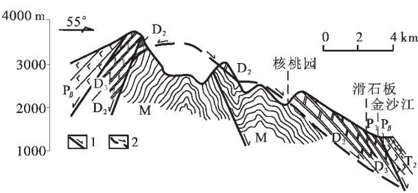
图 6 玉龙—哈巴背斜两翼的拆离构造 [15] M—时代不明变质岩基底;D 2 —中泥盆统大理岩; D 3 —上泥盆统大理岩;P 1 —下二叠统大理岩;P β —二叠纪玄武岩; T 2 —中三叠统砂岩;1—正断层;2—推测拆离断层 Fig.6 Detachment structures in both limbs of the Yulong-Haba anticline [15]
