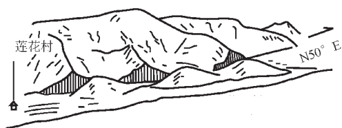
图5 丽江—剑川断裂莲花村剖面图
