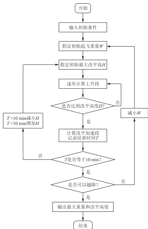
图3 原模型算法计算流程图
