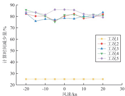
图 5 不同风速和工况的计算时间减少量
