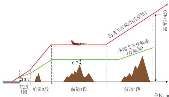
图1 起飞飞行航迹
