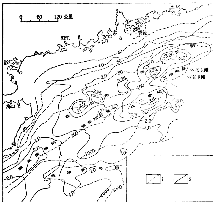
图2 珠江口盆地二级构造分布略图
