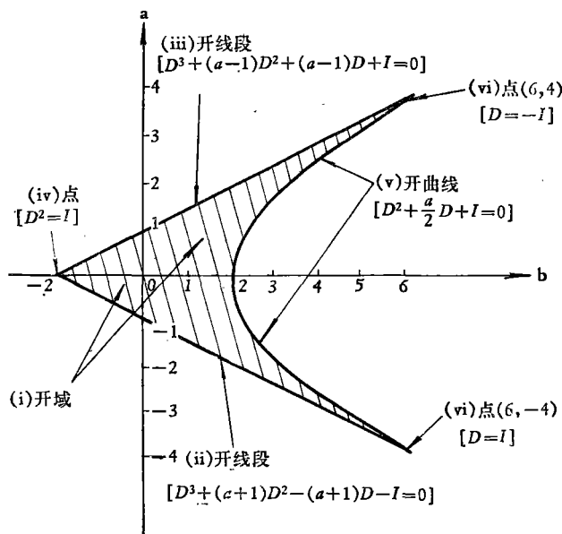
图 1 稳定性图
