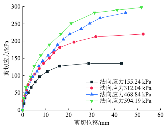
图 11 自反力双剪面大型剪切仪剪切应力-位移曲线
