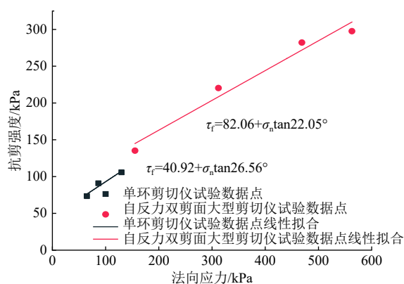
图 12 强度参数拟合对比
