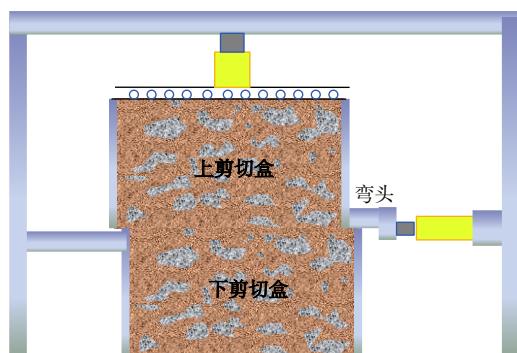
图 2 普通双环直剪仪示意图
