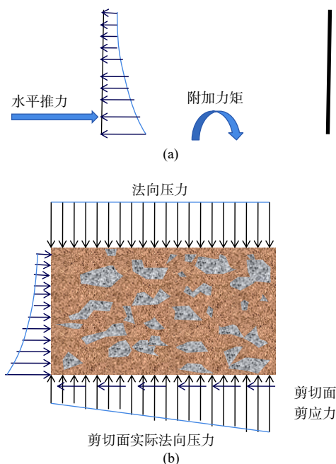
图 5 顶部自由的剪力引起的力偶 (a) 及试样受力简图 (b)
