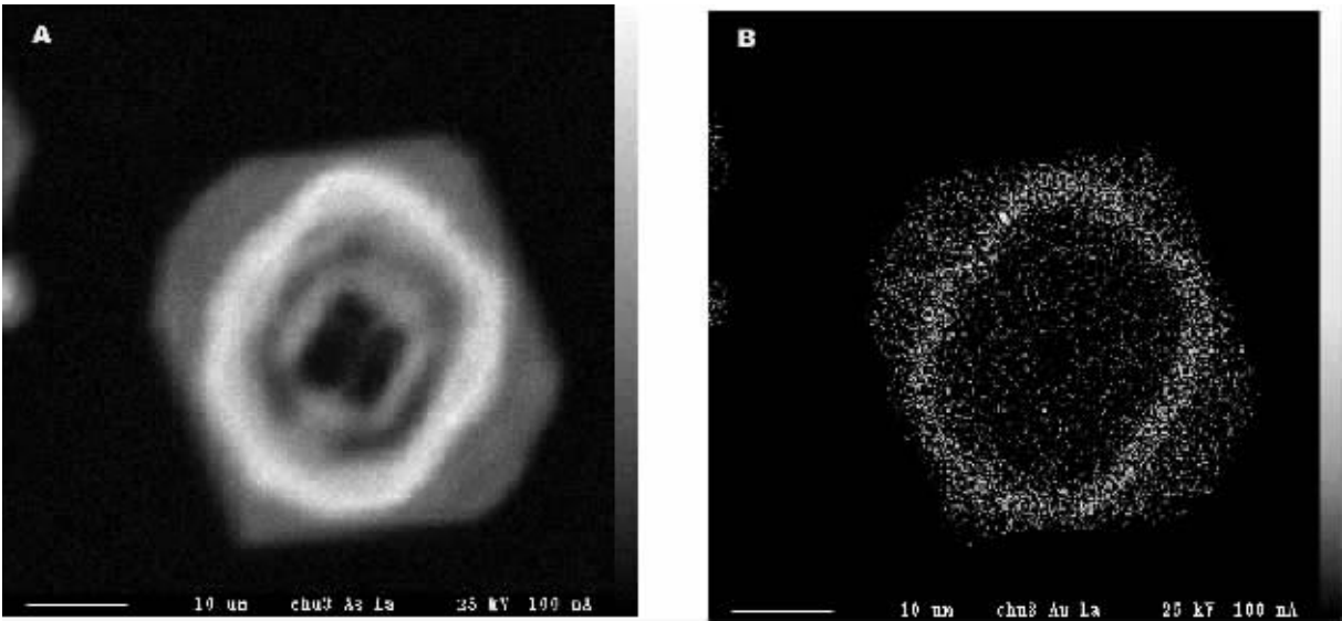
图 5 黄铁矿的电子探针波谱砷 Lα (A)、金 L a(B) 成分扫描图像 Fig.5 Microprobe spectral scan images of the As Lα(A) and Au Lα(B) compositions of pyrite
