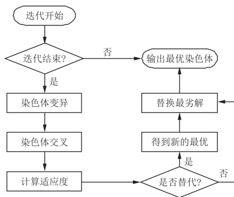
图4 GA迭代过程
