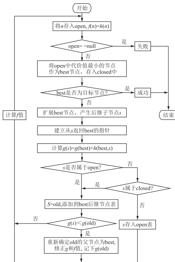
图1 A*算法流程图
