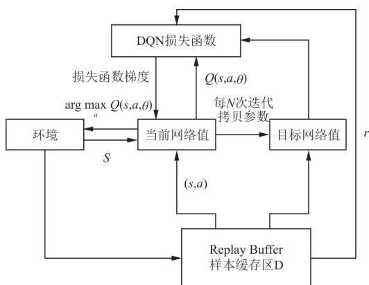
图 7 DQN 算法流程图
