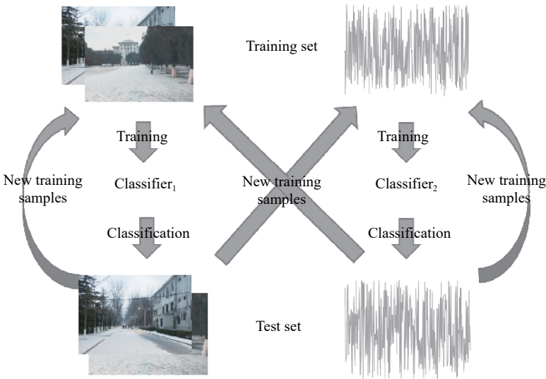
图 4 协同训练
