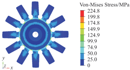
(a) 俯视图
