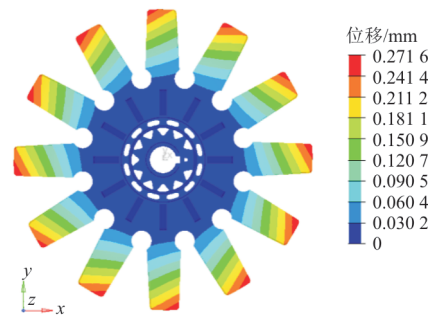
图8 重构模型位移云图
