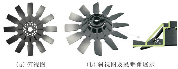
图7 替换件重构模型
