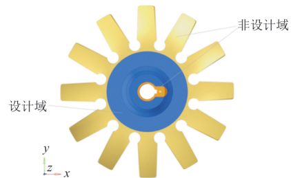
(b) 优化模型设计域
