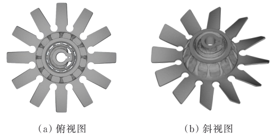
图6 拓扑优化设计构型
