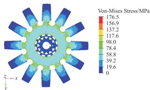
(b) 仰视图
