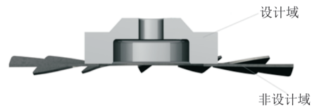
(a) 优化模型剖面图
