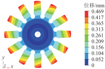
图 2 原件位移云图 Fig. 2 Displacement nephogram of original part
