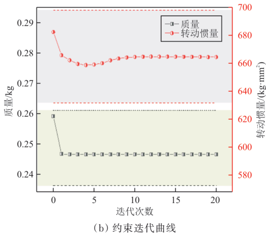
图5 拓扑优化设计迭代曲线
