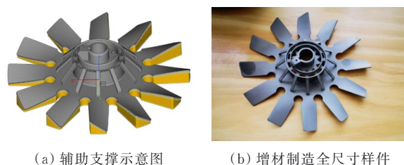
图 10 散热风扇替换件工艺性及样件分析
