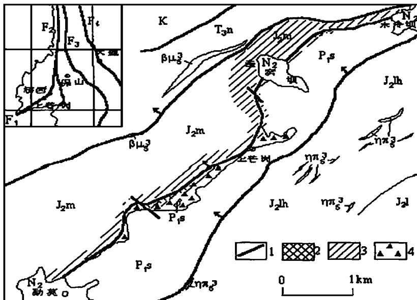
图1 云南上芒岗金矿床矿区地质略图
