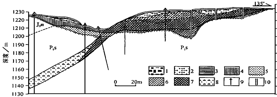
图 3 云南上芒岗金矿床 0 号勘探线剖面图
