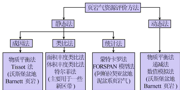
图1 主要页岩气资源评价方法示意图
