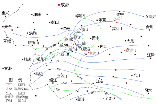
图 3 四川盆地下寒武统筇竹寺组页岩有效厚度等值线图
