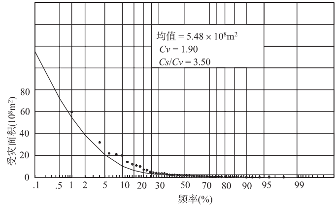
图 6 农田受灾面积频率曲线
