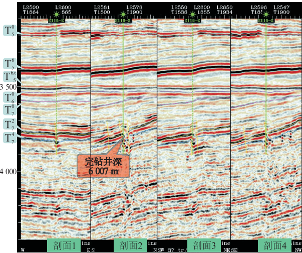
图 1 S116—2 井米字型地震时间偏移剖面 Fig.1 Seismic time migration profile of Well S116—2
