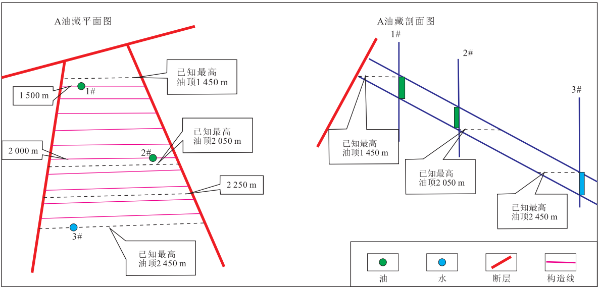
图 1 A 油藏示意图 Fig.1 Diagram of reservoir A
