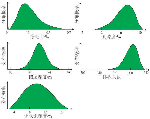
图 4 概率法储量估算中主要估算参数的常用函数形态 Fig. 4 Usual function forms of major estimation parameters in probabilistic method
