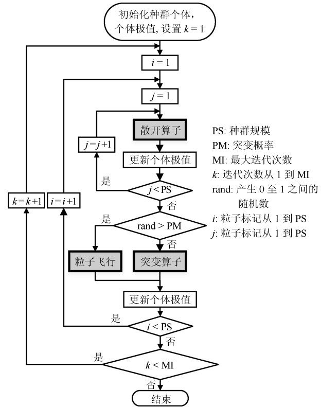
图 5 算法流程图 Fig. 5 Algorithm flowchart
