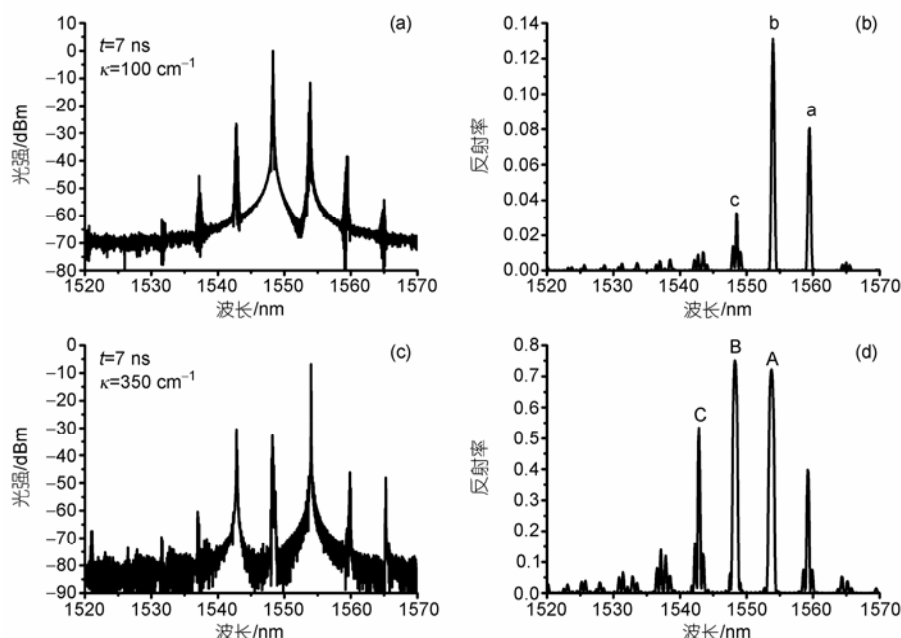
图 5 前向切换过程中模式竞争现象及相应的 SGDBR 反射谱乘积图
