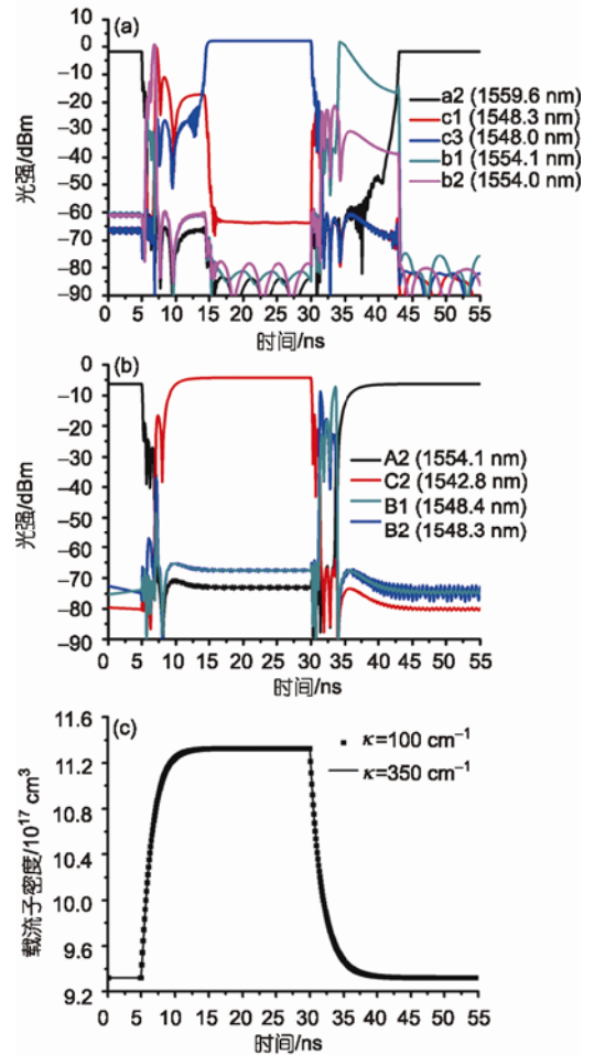
图 4 不同 \kappa 值下模式强度及 RSG 中载流子密度随时间的变化
