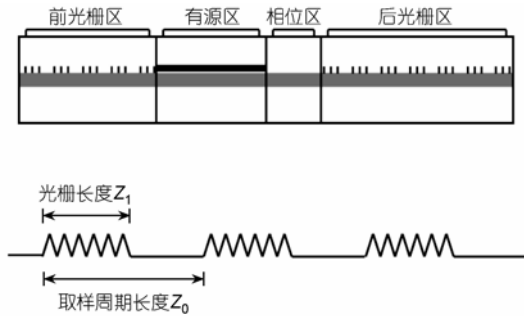
图1 四段式SGDBR可调谐半导体激光器结构示意图
