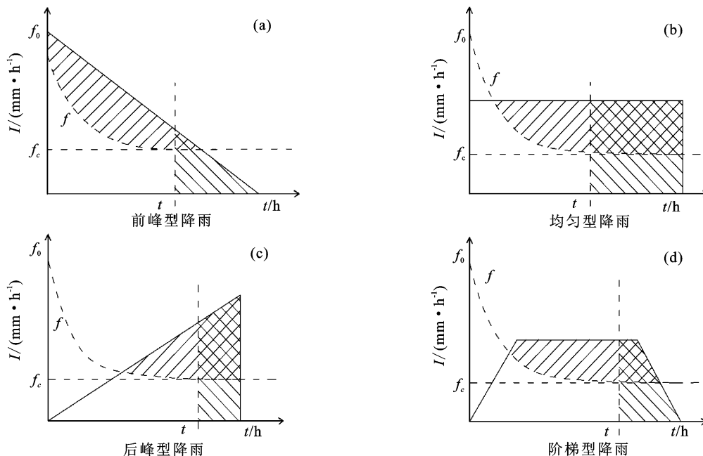
图 3 降雨雨型
