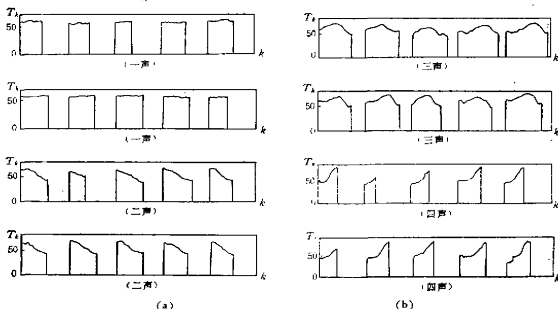
图 5 基音轮廓的检测结果
