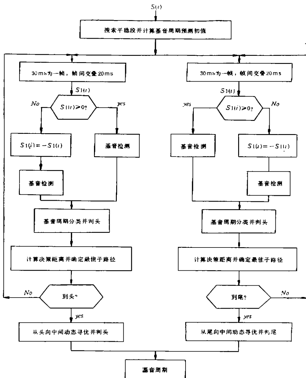
图2 基音检测器框图
