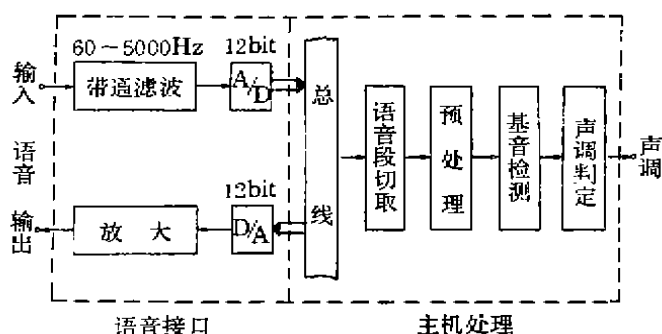
图1 系统框图
