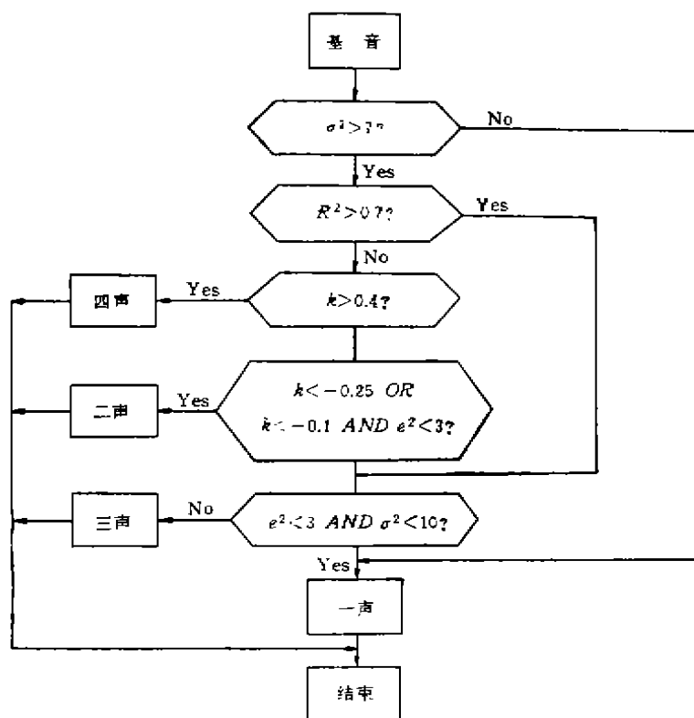
图8 声调判定框图
