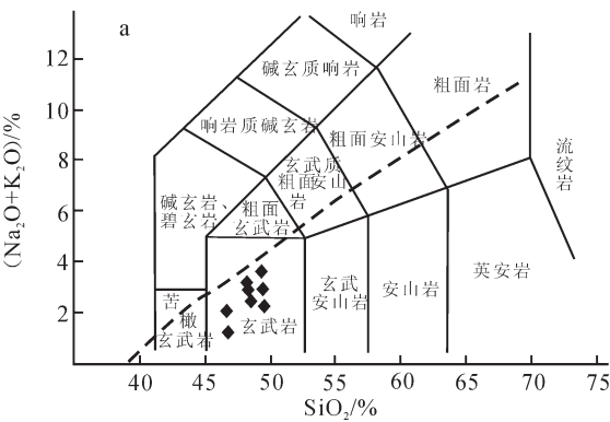
图 7 香山群辉绿岩 TAS 分类图和 Nb/Y-Zr/TiO 2 图解 Fig.7 TAS classification and Nb/Y-Zr/TiO 2 diagrams of diabase in the Xiangshan Group
