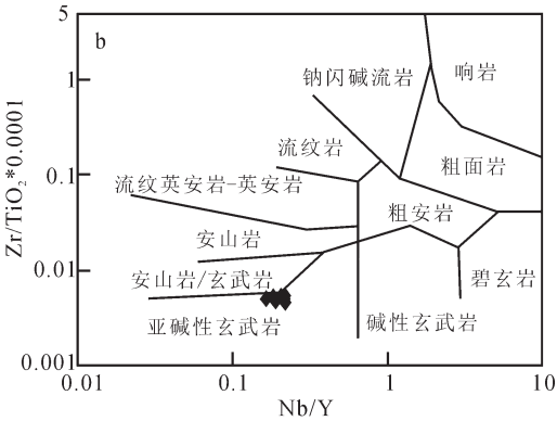
图 7 香山群辉绿岩 TAS 分类图和 Nb/Y-Zr/TiO 2 图解 Fig.7 TAS classification and Nb/Y-Zr/TiO 2 diagrams of diabase in the Xiangshan Group
