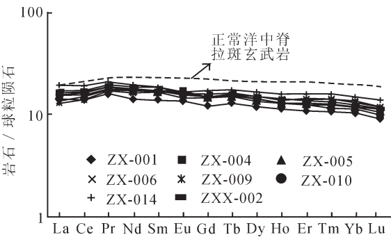
图 8 香山群辉绿岩球粒陨石标准化 REE 型式(球粒陨石标准化数据据 Boynton, 1984) Fig.8 Chondrite-normalized REE patterns of diabase in the Xiangshan Group
