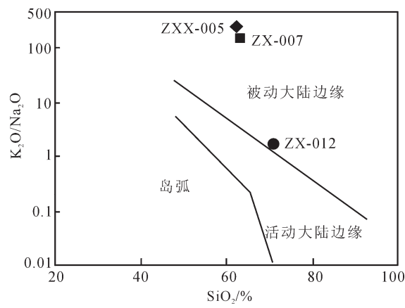
图 5 碎屑岩主量元素对构造背景的指示 (底图据 Roser 和 Korsch, 1986)
