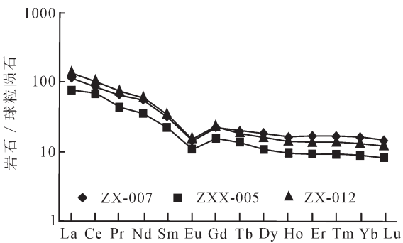
图 6 碎屑岩球粒陨石标准化 REE 型式 (球粒陨石标准化数据据 Boynton, 1984) Fig.6 Chondrite-normalized REE patterns of clastic rocks in the Xiangshan Group
