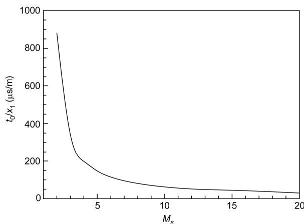
图 2 直通型激波风洞试验时间
