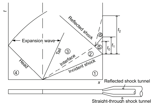
图 1 激波风洞波图. t_0 : 直通型激波风洞试验时间, t_1 : 反射型激波风洞试验时间(远离缝合), t_2 : 反射型激波风洞试验时间(缝合分界面)
