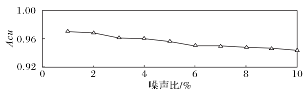
图 5 LSTM 在不同噪声百分比下预测拟合数据的 Acu
