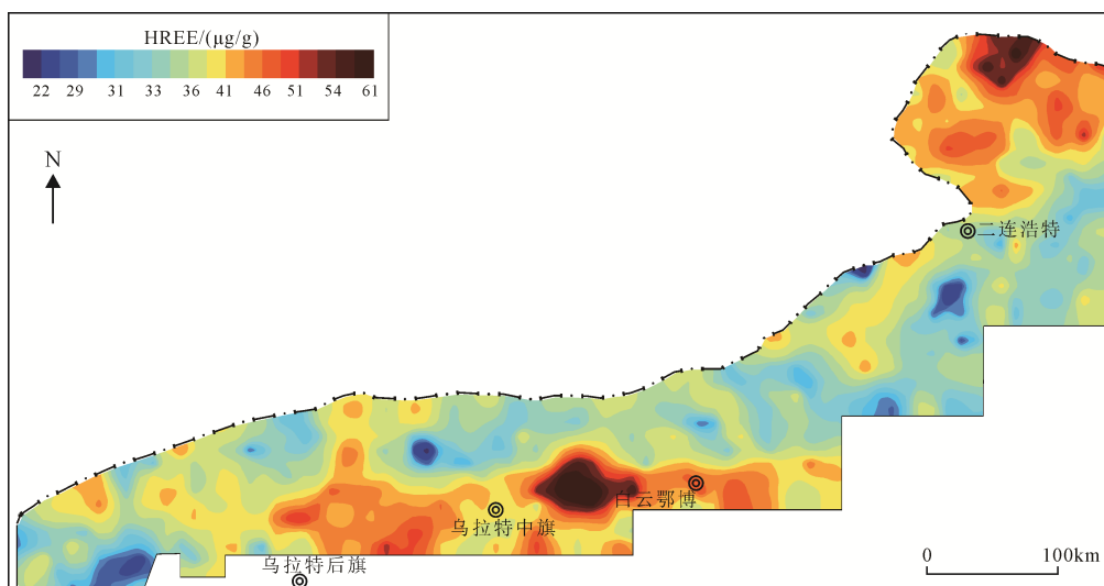
图 5 白云鄂博及邻区重稀土地球化学图
