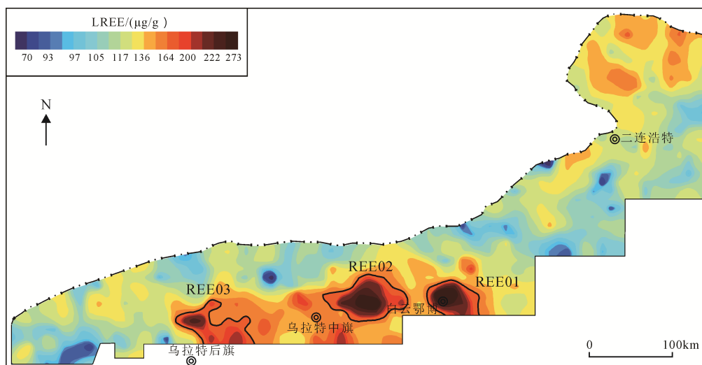
图 4 白云鄂博及邻区轻稀土地球化学图
