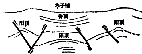
图3 雷音铺——七里峡之间地震示意剖面(据四川石油管理局地调处)
