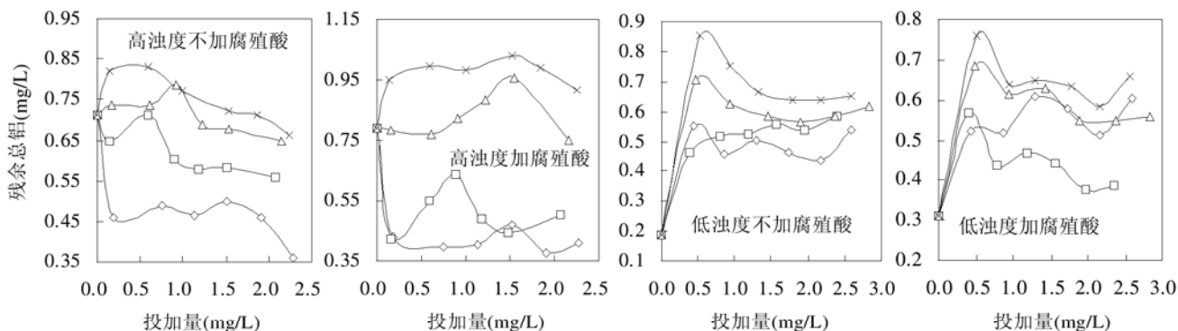
图 3 铝系混凝剂在不同混凝体系中的残余总铝
