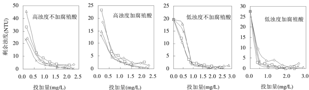
图 2 铝系混凝剂在不同混凝体系中的除浊效果
