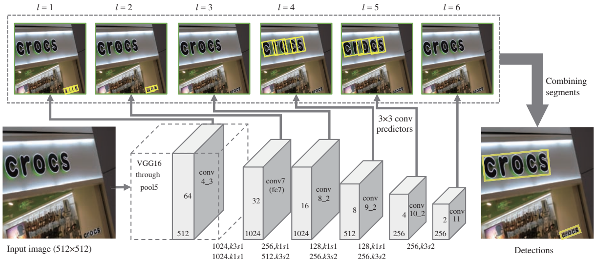
图 3 (网络版彩图) SegLink 的网络框架示意图 [20] . 特征层之间的卷积滤波器用“(滤波器维度), k (卷积核尺寸), s (卷积步长)”来表示. 首先, 文字片段 (黄色包围盒) 及其连接关系 (未显示) 通过多个特征层预测 (以 l 为编号); 然后, 通过一个结合算法将它们联结为一个单词的包围盒
