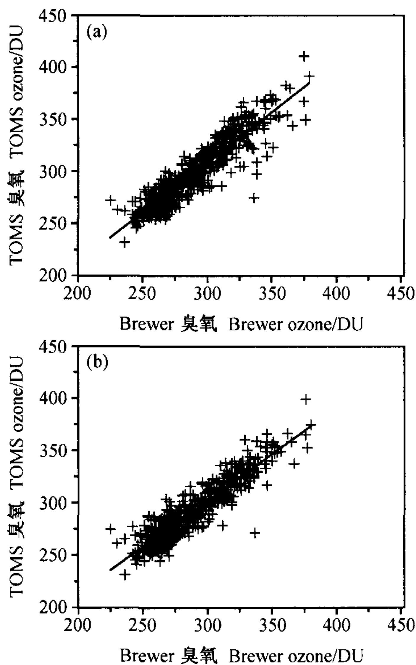
图 2 Brewer 数据与 TOMS 版本 7 (a) 和版本 8 (b) 数据的相关分析
