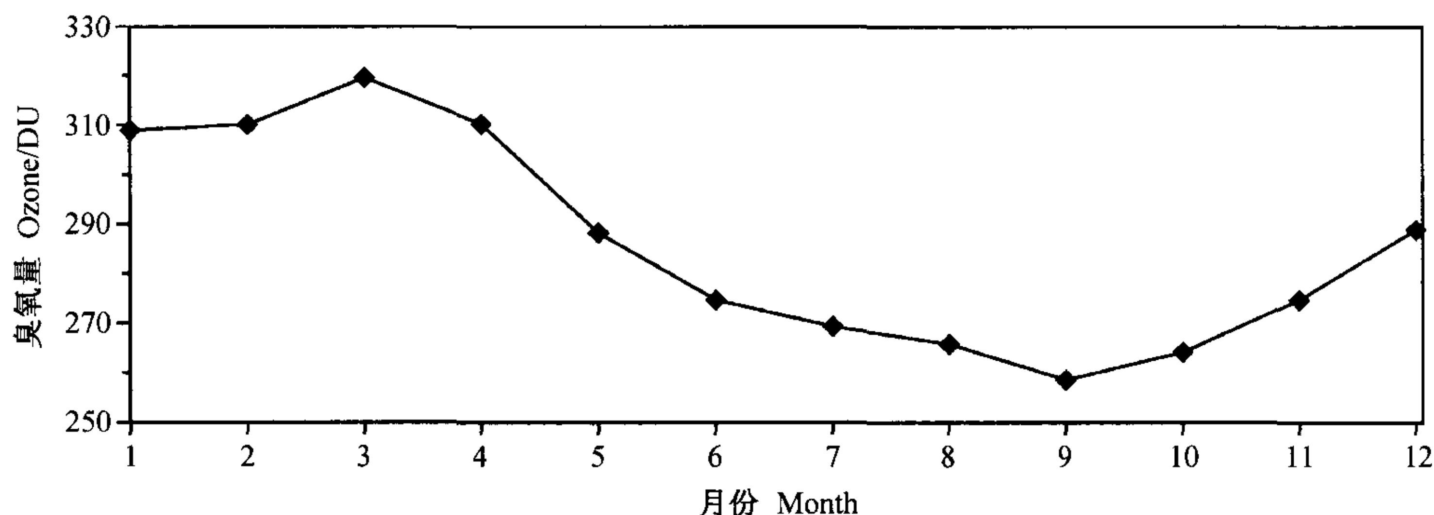
图4 瓦里关地区臭氧总量的季节变化
