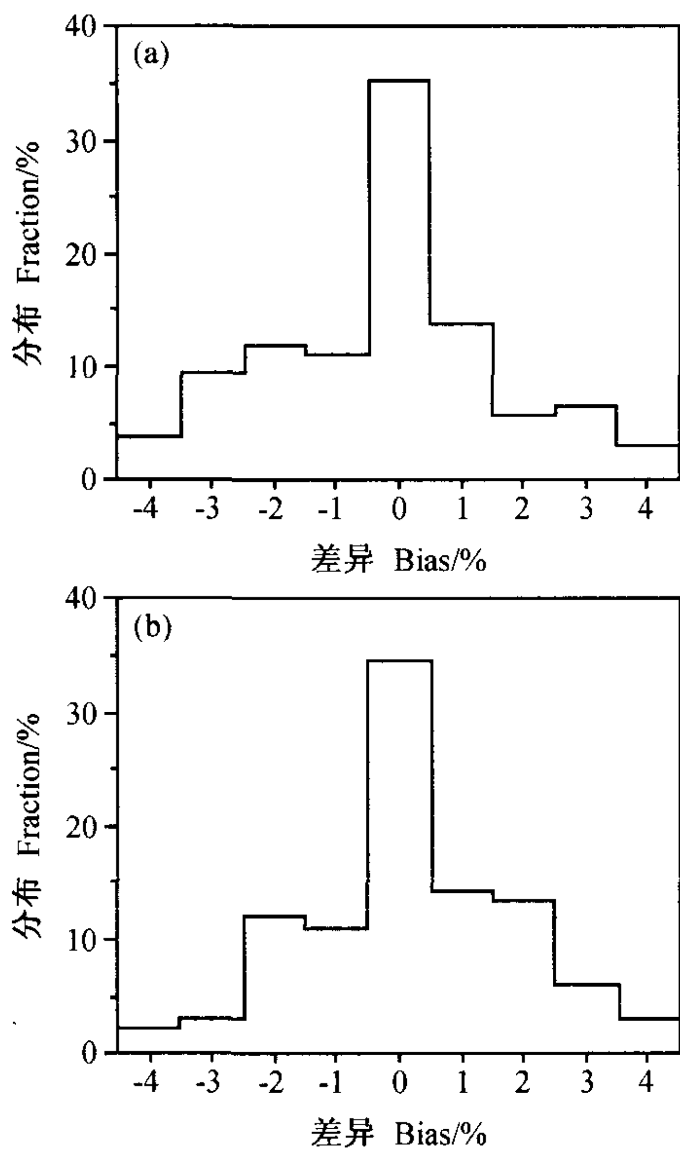
图 1 Brewer 数据与 TOMS 版本 7 (a) 和版本 8 (b) 数据的差异
