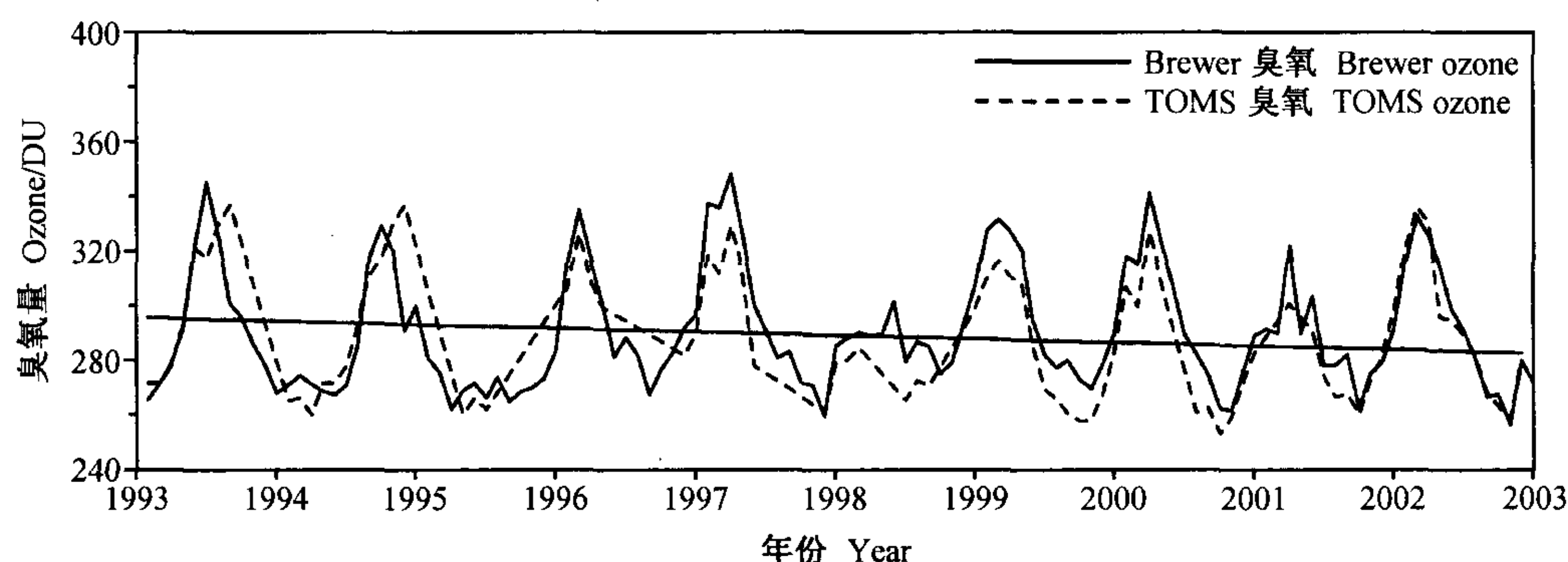
图 3 瓦里关地区臭氧总量的月平均变化（线性拟合趋势： y = -0.106x + 295.51 ）
