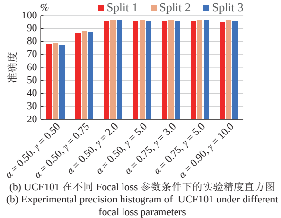
图8 不同 Focal loss 参数条件下实验精度直方图
