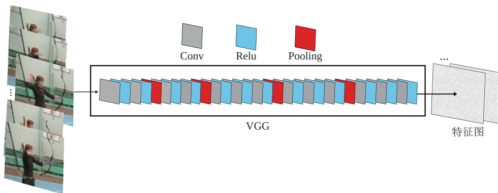
图 1 VGG 特征提取器
