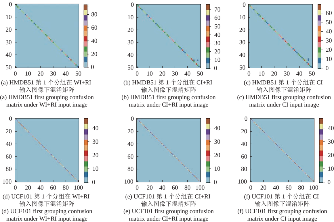
图 9 混淆矩阵 Fig.9 Confusion matrix
