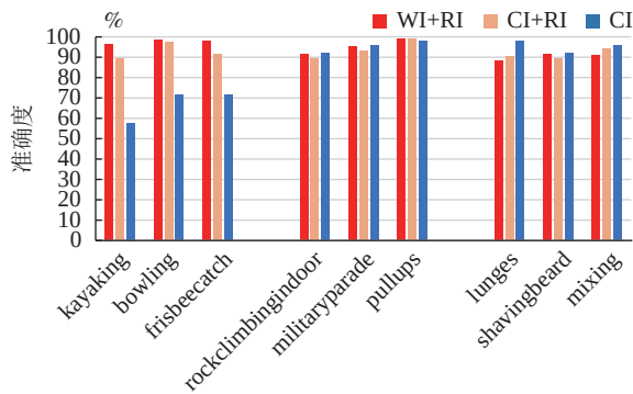
(a) UCF101 在不同的输入图像下部分类别精度对比 (a) UCF101 partial category accuracy comparison under different input images
