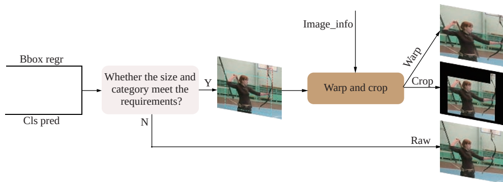
图 4 目标区域获取与图像变换
