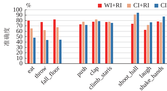
(b) HMDB51 在不同的输入图像下部分类别精度对比 (b) HMDB51 partial category accuracy comparison under different input images
