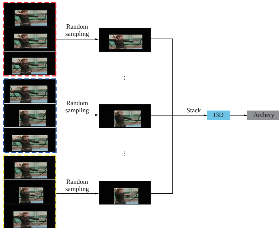
图 5 视频分段随机采样
