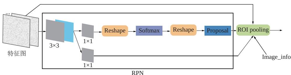
图 2 区域候选网络
