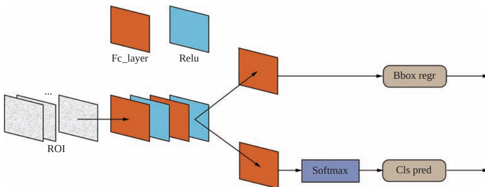
图 3 边框回归与类别预测
