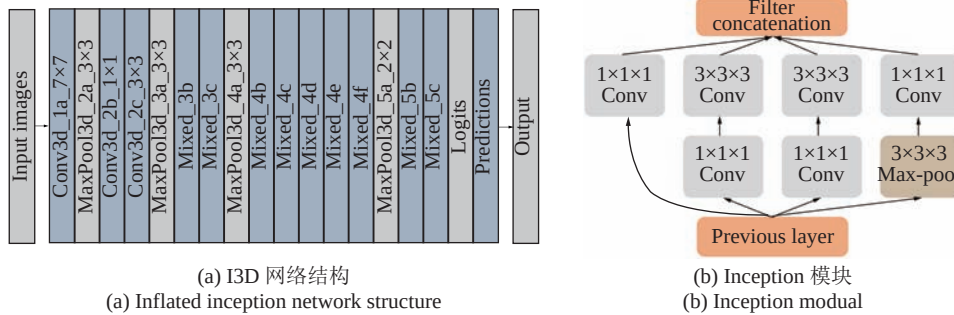
图 6 I3D 网络
