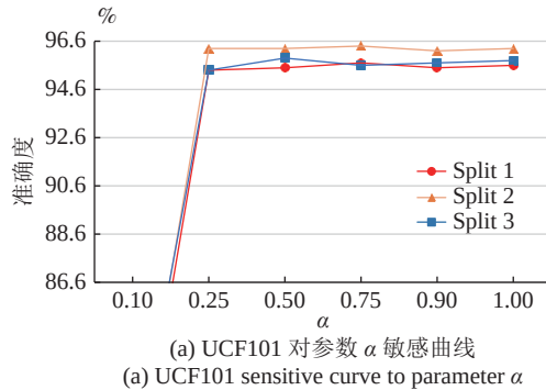
图7 Focal loss 参数 \alpha 敏感曲线
